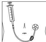
Magensonde (PEG-Sonde)
