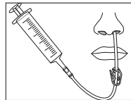
Nasensonde (NG-Sonde)
